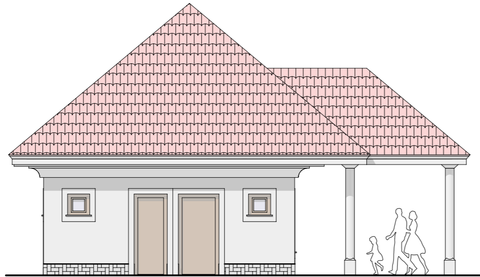
SEVERO-VZHODNA FASADA
