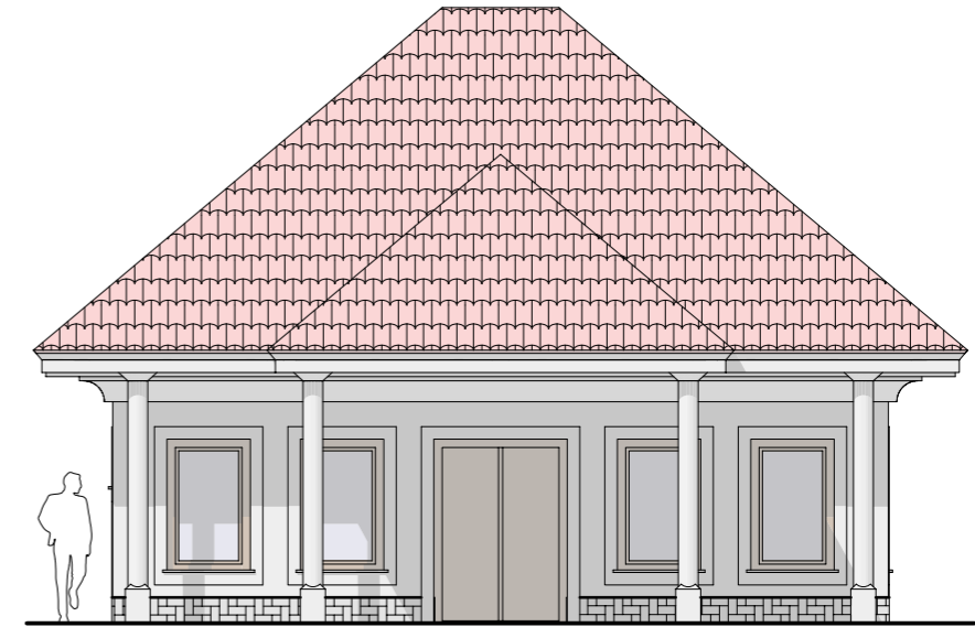
SEVERO-ZAHODNA FASADA
